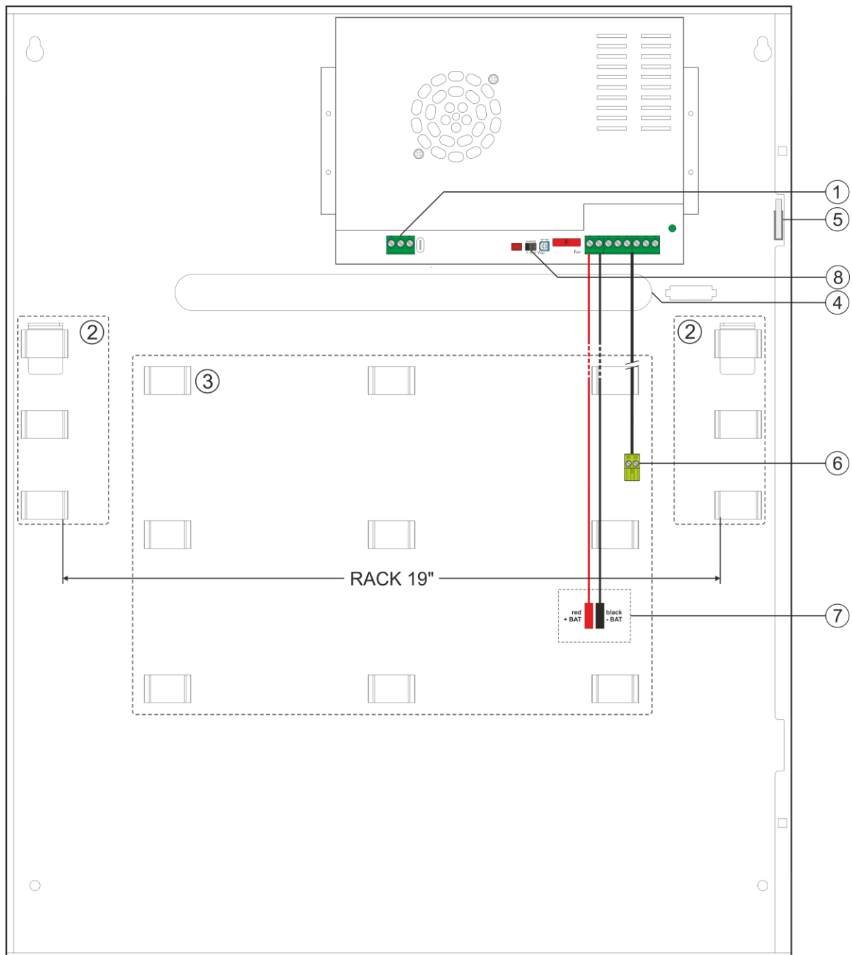
Rys.3. Widok zasilacza.
