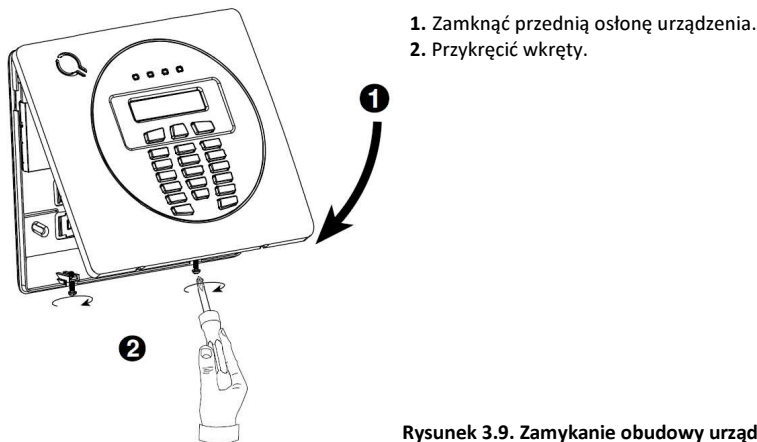
Rysunek 3.9. Zamykanie obudowy urządzenia
